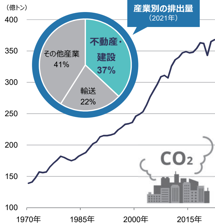
世界の二酸化炭素排出量の推移（1970年～2022年）
